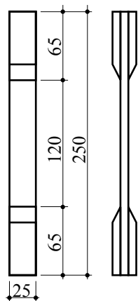
Fig.2 JIS K 7054
