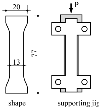
Fig.3 JIS K 7056
